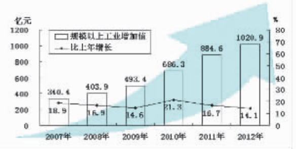
保定市2007-2012年规模以上工业增加值及其增速图表
