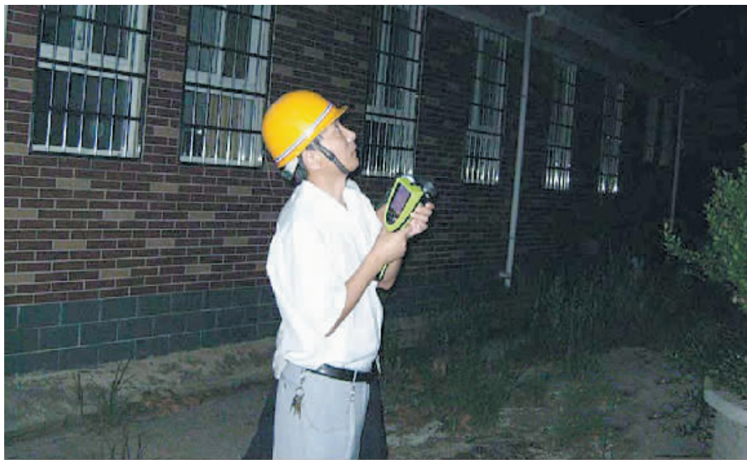
7月16日晚用电高峰时段,光山县电业局线路工区组织人员对110千伏光山变电站、紫水变电站的进出线连接点线夹以及35千伏线路进行了夜巡测温,旨在及时发现并消除输电线路安全隐患,确保迎峰度夏可靠供电。张磊 向金旗 摄
