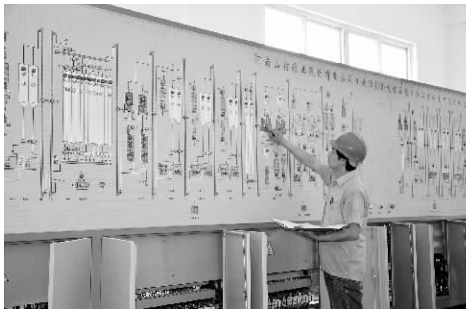
近日,武汉良友机电公司工程师在对河南山信粮业有限公司新组装的自动化控制系统进行检测。位于商城县产业集聚区的河南山信粮业有限公司,是一家集粮食收购、加工、仓储、销售于一体的大型民营企业,其新安装的日处理1000吨稻谷精米加工中心生产线自动化控制系统,将于7月份正式投入使用。
