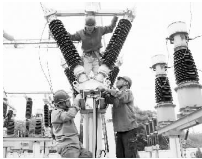
信阳供电公司秋季检修工作于近日全面铺开,确保迎峰度冬可靠供电。图为10月11日,该公司工作人员对110千伏侯家湾变电站更换隔离刀闸。 王强 刘威 摄
